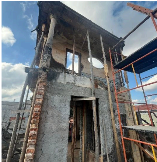
Escoramento para reforço estrutural no pavimento superior. Autoria: Eduardo Santos Data: 10/06/2025
