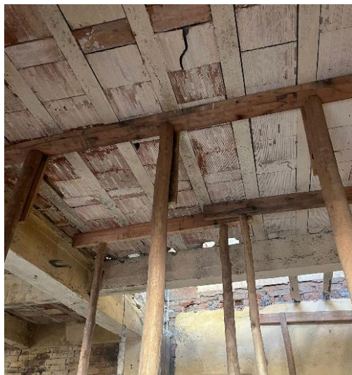
Escoramento para execução de reforço estrutural.
